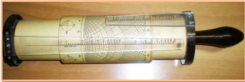
Regolo cilindrico “Stanley” per operazioni sui numeri complessi
