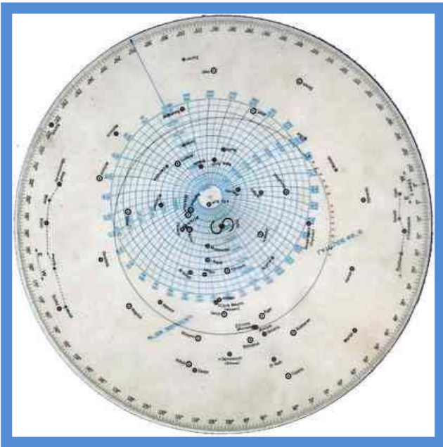
Regolo circolare (per la navigazione astronomica)
