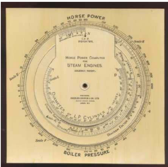
Regolo calcolatore (per Boiler Pressure)
