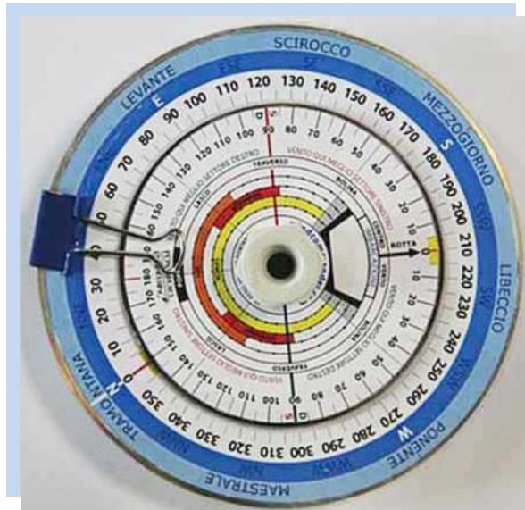
Regolo calcolatore dei venti
