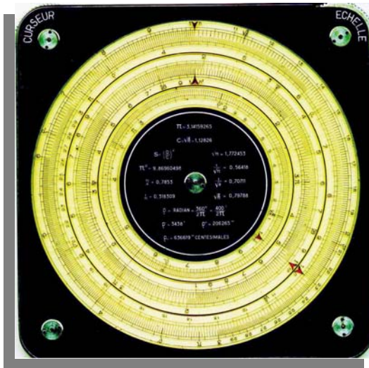
Regolo circolare “Roplex” Cursore e scorrevole manovrati con meccanismi micrometrici
